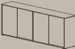
Buffet 4/A 4/D Sideboard Buffet 4/P L 202 W 48 H 83
